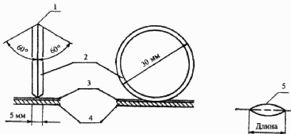
1 — острый край; 2 — индентор; 3 — покрытие; 4 — основание; 5 — форма отпечатка
