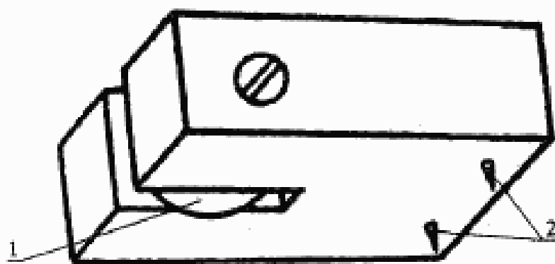
1 — индентор; 2 — опоры
